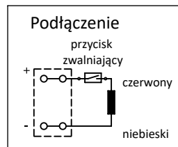
Przycisk zwalniający na boku Wejście kabla od dołu
