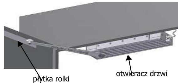
Rysunek 10. Widok od przodu – drzwi „lewe”
