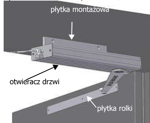
Rysunek 11. Widok od tyłu – drzwi „lewe”
