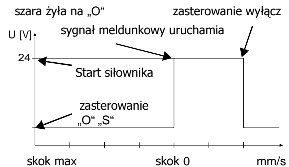
Rysunek 2. Wykres sygnału meldunkowego w kierunku ZAMKNIJ
